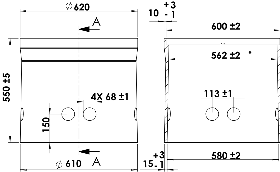
SECTION A-A SCALE 1 : 9
